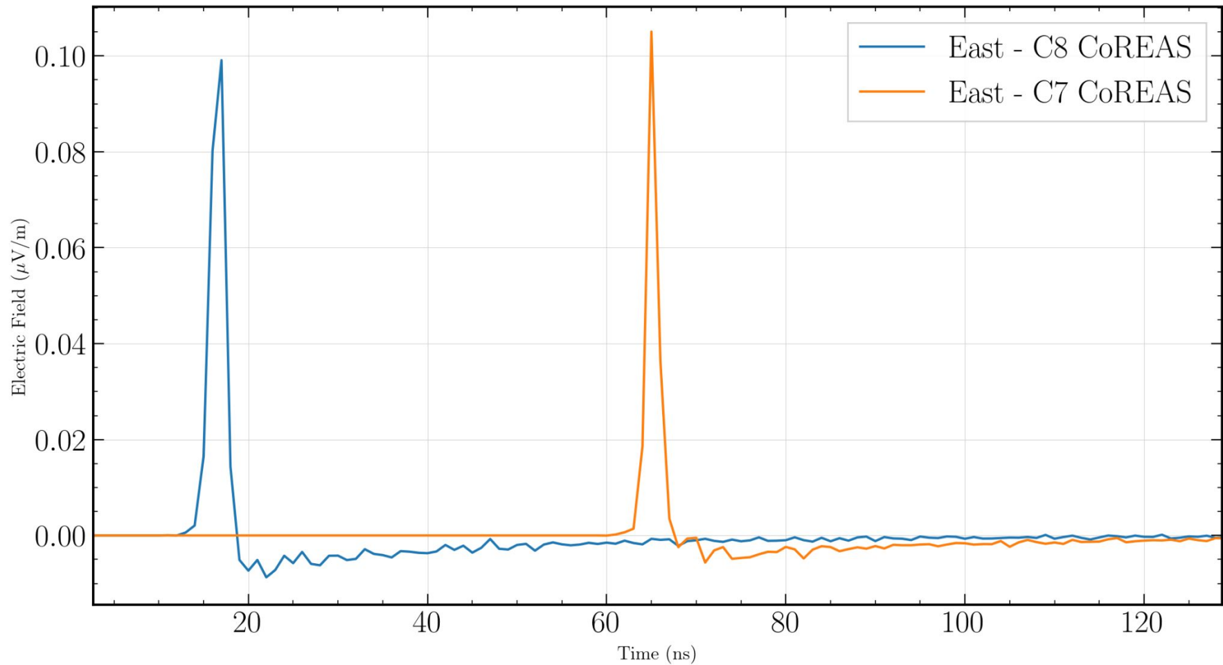
Antenna 200 m - CoREAS -
