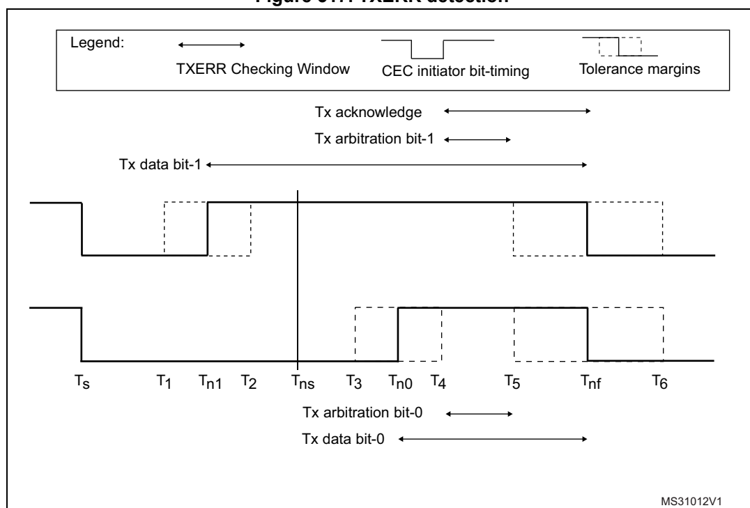
Figure 517. TXERR detection
