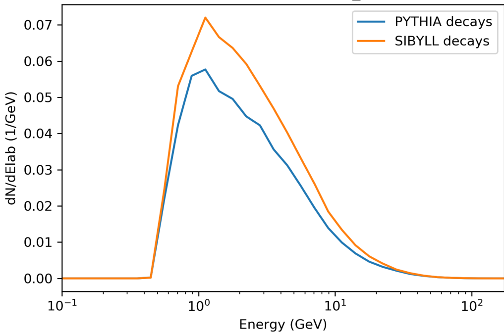
158 GeV, SIBYLL23C, PDG_ID=310
