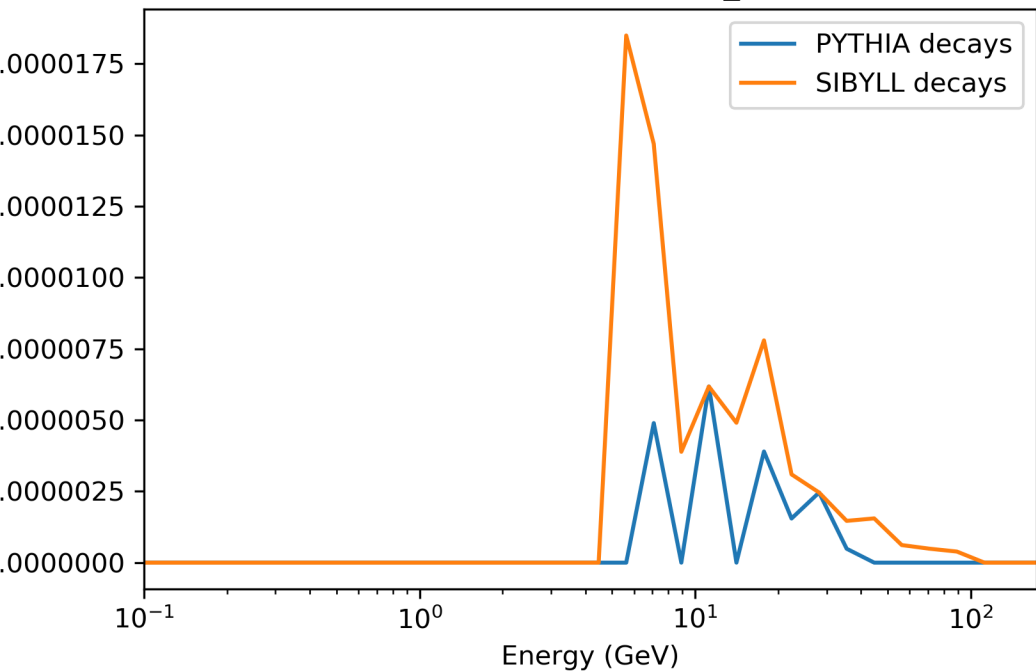
158 GeV, SIBYLL23C, PDG_ID=-421
