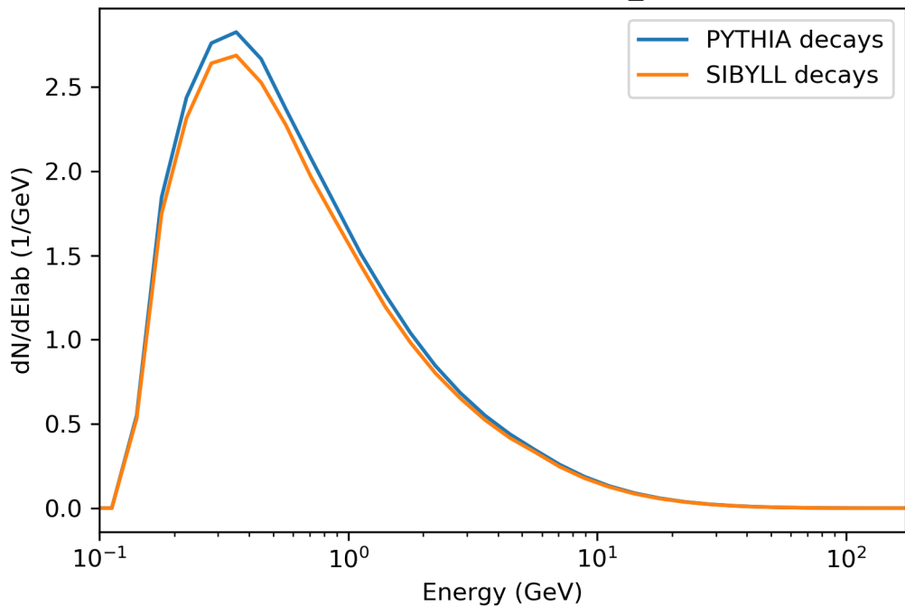
158 GeV, SIBYLL23C, PDG_ID=211
