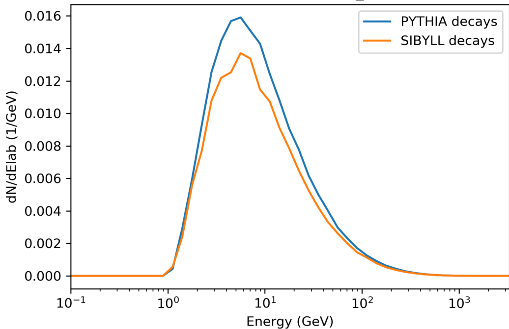
3000 GeV, SIBYLL23C, PDG_ID=-2212
