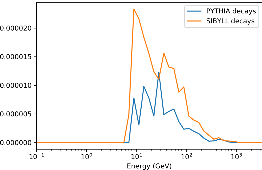
3000 GeV, SIBYLL23C, PDG_ID=-431
