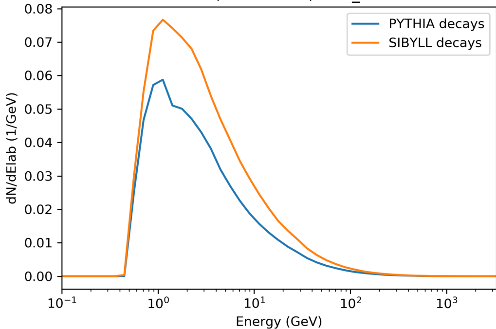
3000 GeV, SIBYLL23C, PDG_ID=310
