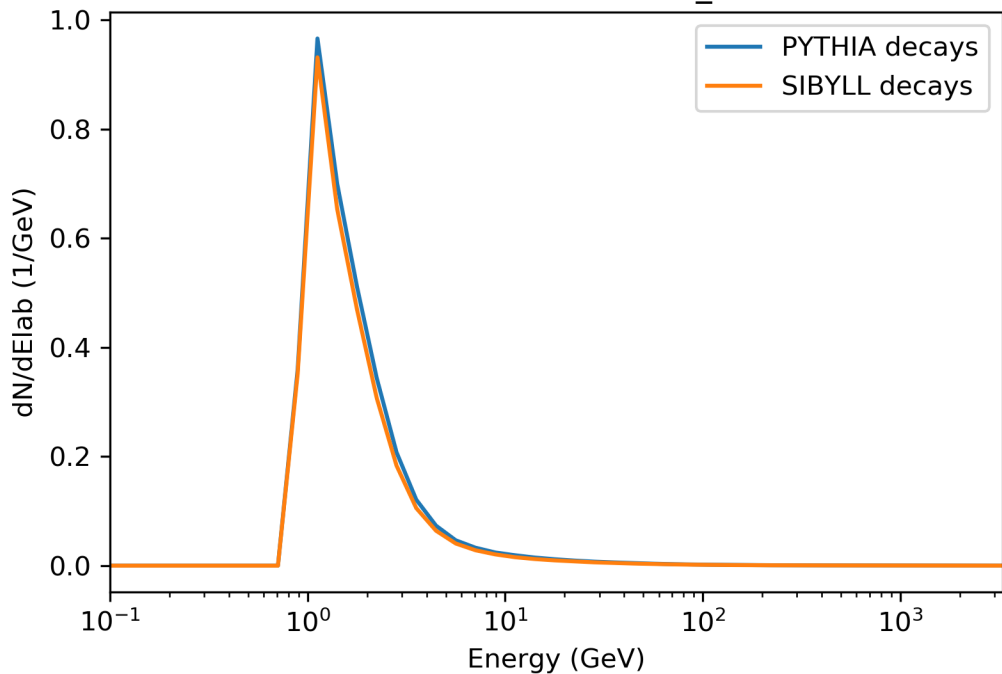
3000 GeV, SIBYLL23C, PDG_ID=2112
