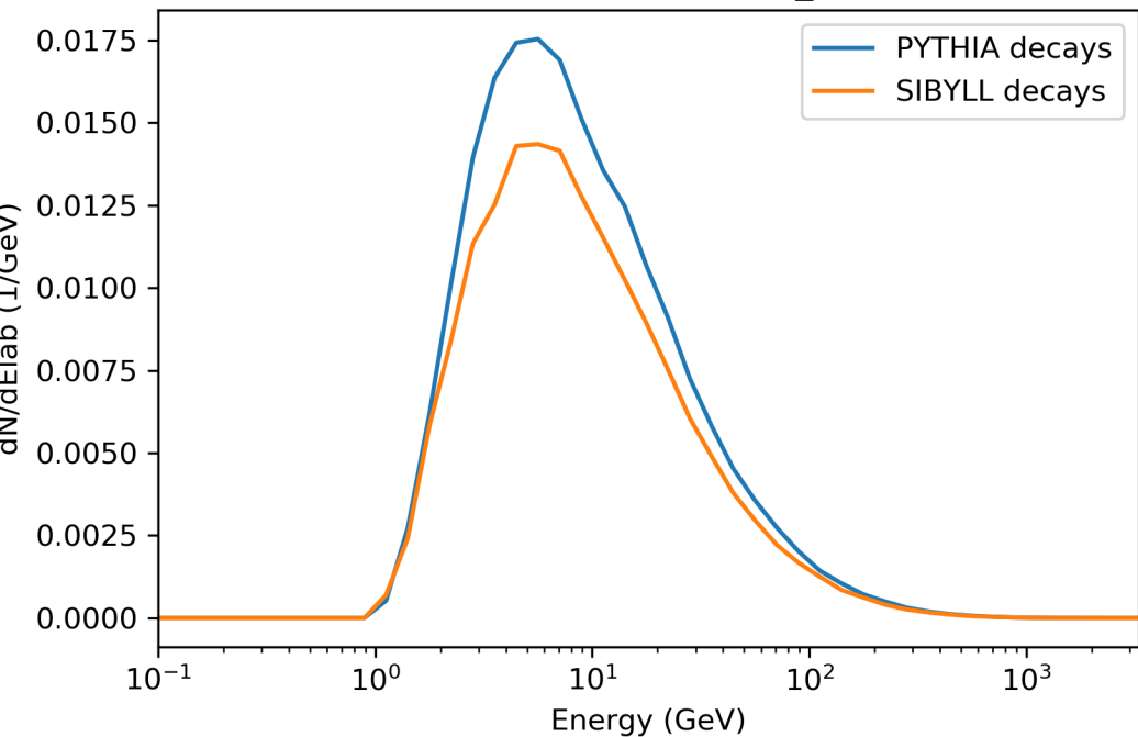
3000 GeV, SIBYLL23C, PDG_ID=-2112
