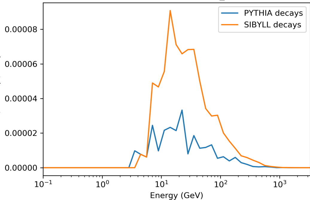
3000 GeV, SIBYLL23C, PDG_ID=-421
