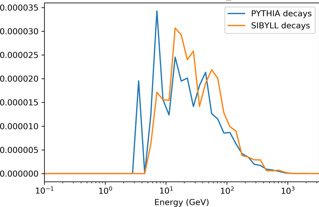
3000 GeV, SIBYLL23C, PDG_ID=-411
