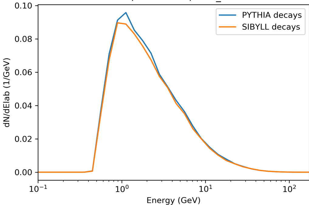
158 GeV, SIBYLL23C, PDG_ID=321
