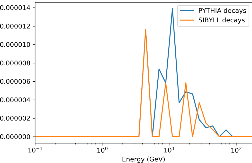
158 GeV, SIBYLL23C, PDG_ID=-411
